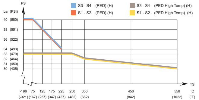
AlfaNova XP27- Graphique de pression / température homologué DESP
