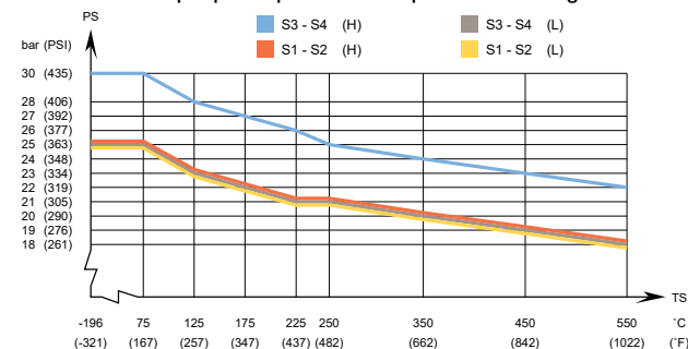
AlfaNova 27 – Graphique de pression / température homologué DESP
