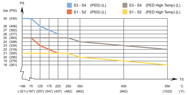
AlfaNova HP 27 - Graphique de pression / température homologué haute température DESP
