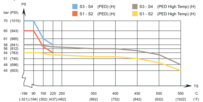
AlfaNova XP27 - Graphique de pression / température homologué haute température DESP
