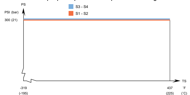
AlfaNova 14 – Graphique de pression / température homologué UL
