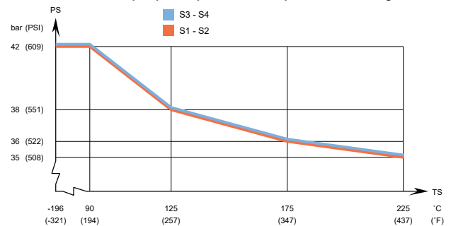
AlfaNova HP 14 - Graphique de pression / température homologué DESP
