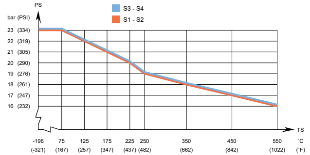
AlfaNova 14 – Graphique de pression / température agréé DESP
